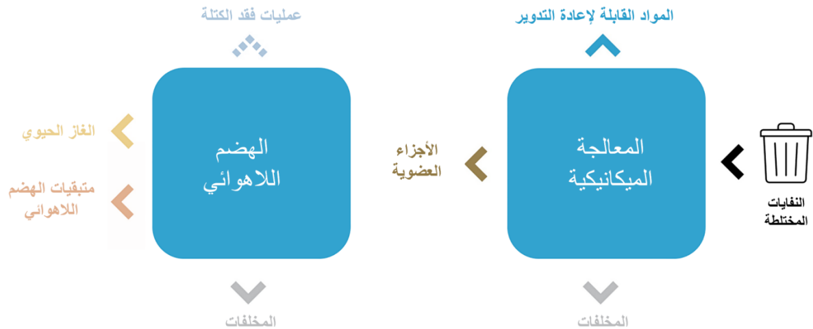
الشكل 0-1: مخطط عملية سير المعالجة الميكانيكية البيولوجية باستخدام الهضم اللاهوائي.
