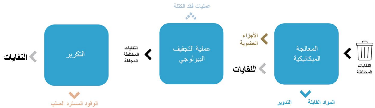
الشكل 6-0: مخطط عملية سير التكرير للمعالجة الميكانيكية البيولوجية - الخيار الأول
