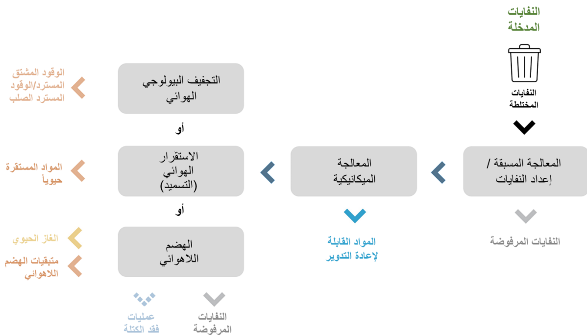
الشكل 0-4: مخطط سير عملية المعالجة الميكانيكية البيولوجية.
