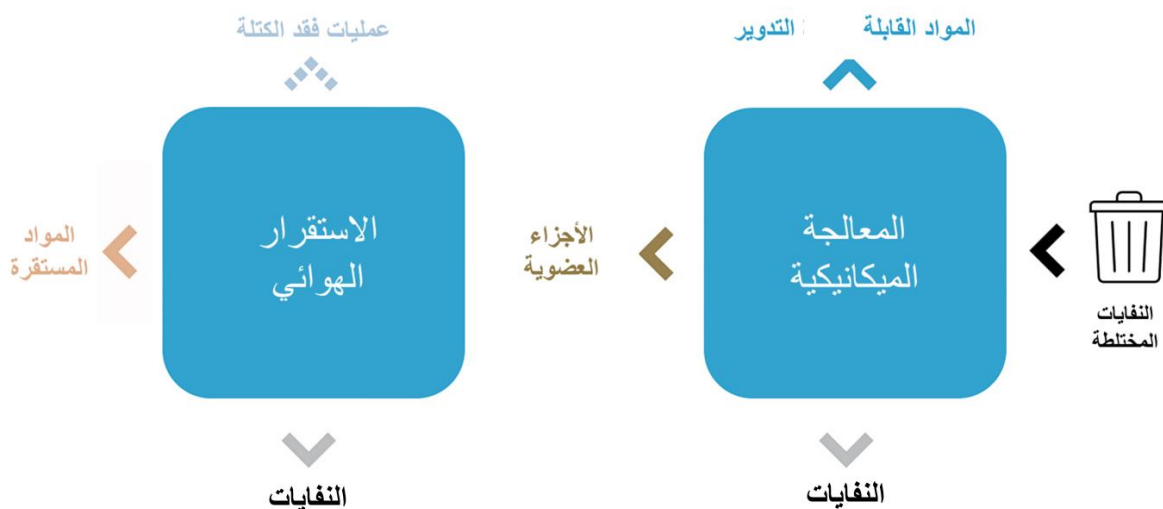
الشكل 6-0: مخطط عملية سير المعالجة الميكانيكية البيولوجية باستخدام الاستقرار الهوائي.
