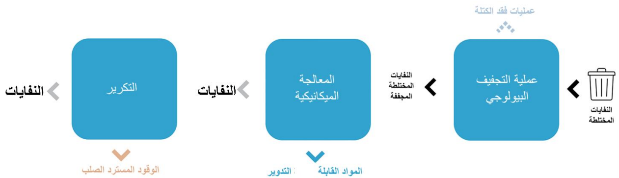
الشكل 6-0: مخطط عملية سير التكرير للمعالجة الميكانيكية البيولوجية - الخيار الثاني.
