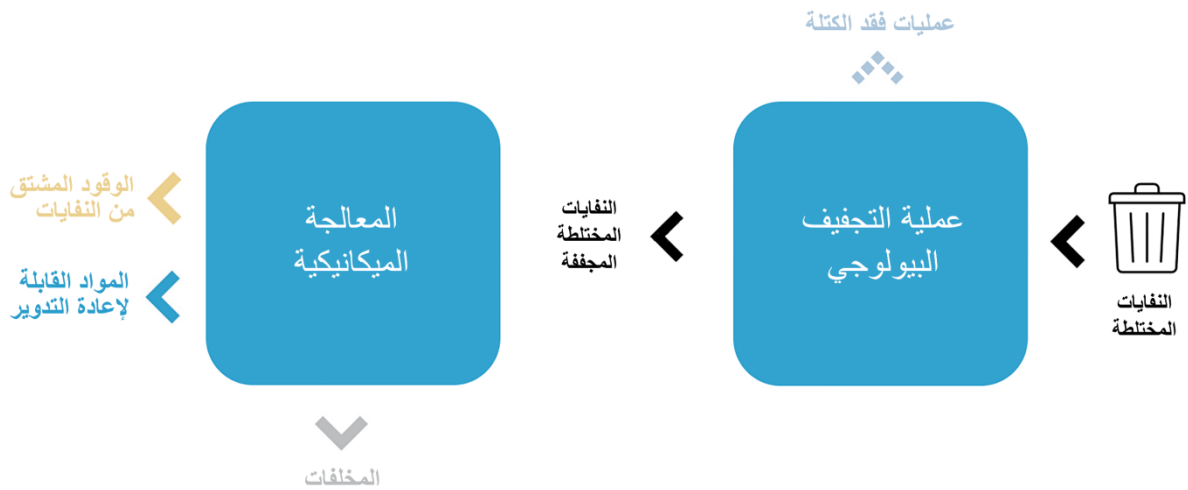
الشكل 0-6: مخطط عملية سير التجفيف البيولوجي للمعالجة الميكانيكية البيولوجية - الخيار الثاني.
