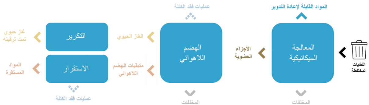
الشكل 0-6: مخطط عملية سير المعالجة الميكانيكية البيولوجية باستخدام الاستقرار الهوائي.
